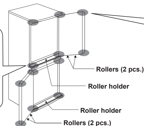
Rollers (2 pcs.)
