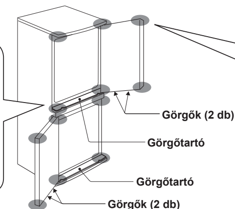
Görgők (2 db)
