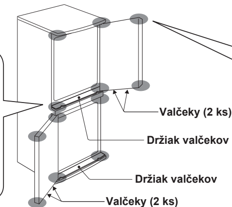
Mechanická časť
