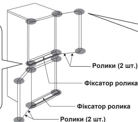
Ролики (2 шт.)
